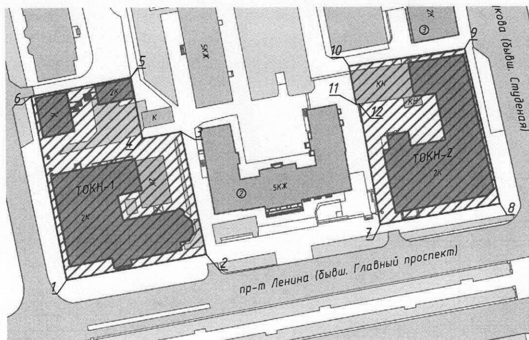
Карта (схема) границ территории Объекта
